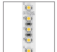
Duratape ES Indoor 4.4W / 2200K / 84CRI
